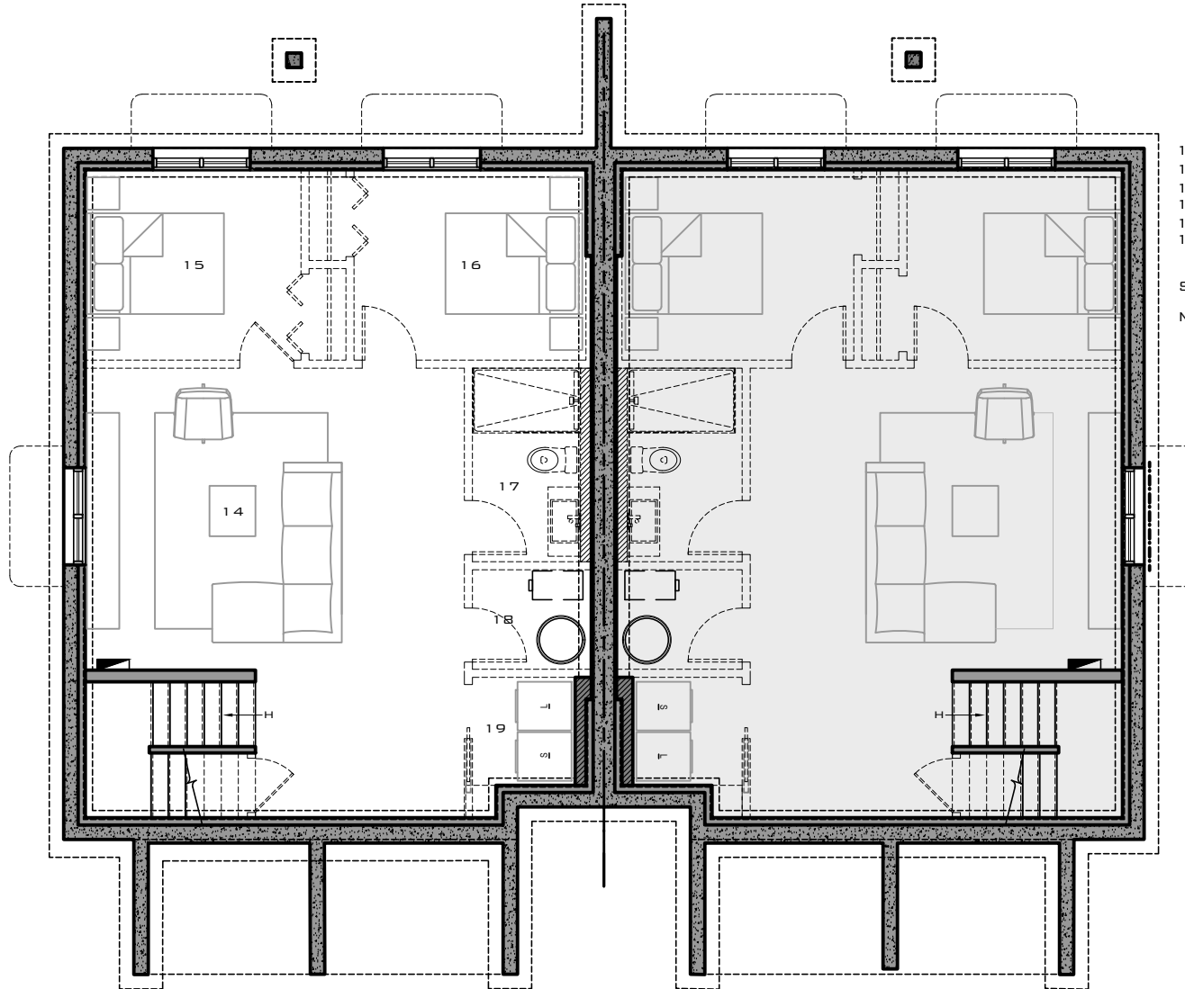
PLAN D'AMÉNAGEMENT - SOUS-SOL
