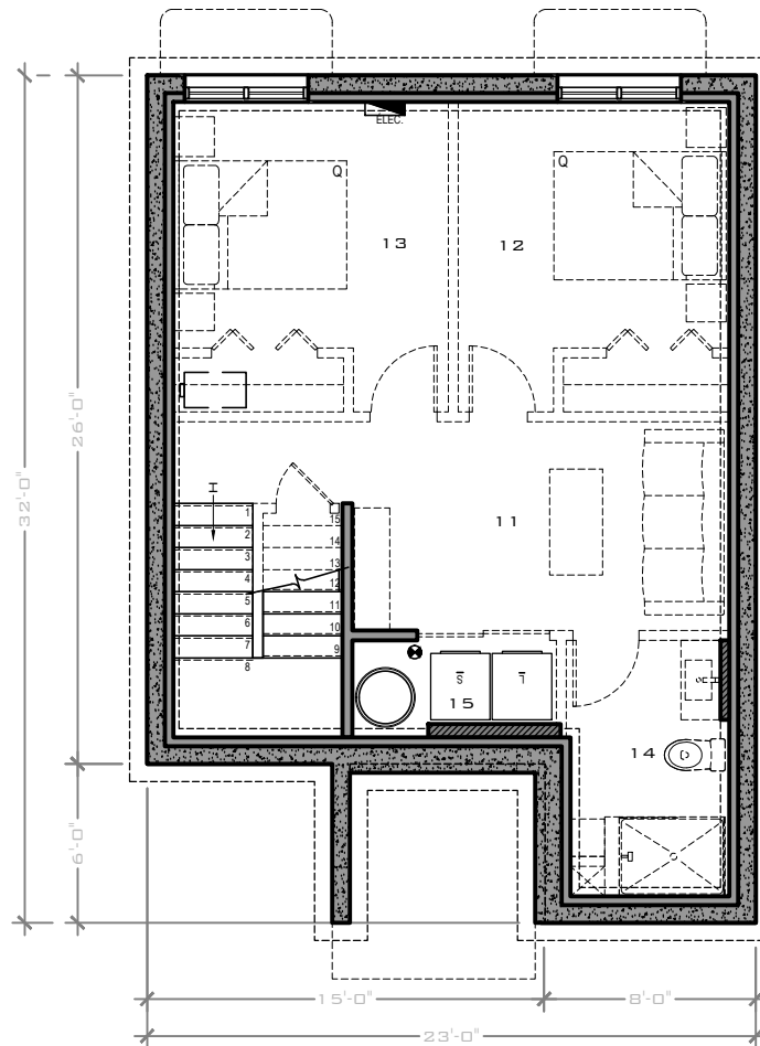
PLAN D'AMÉNAGEMENT - SOUS-SOL
