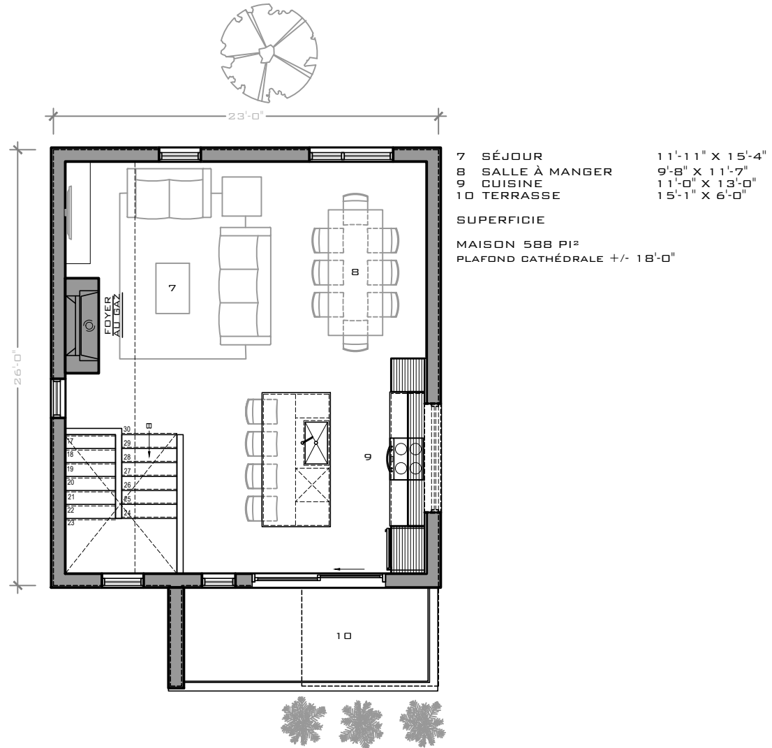
PLAN D'AMÉNAGEMENT - ÉTAGE
