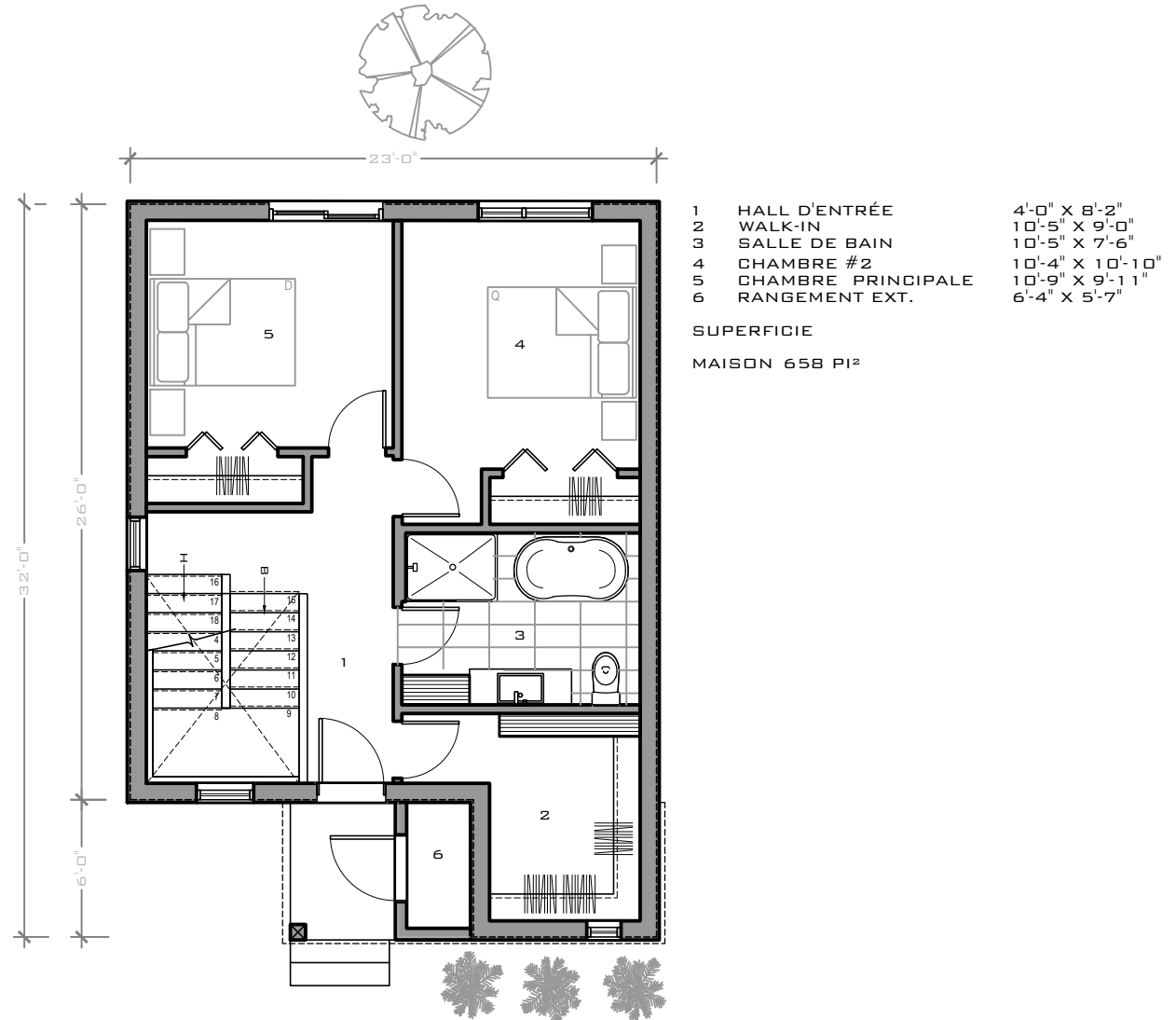
PLAN D'AMÉNAGEMENT - REZ-DE-CHAUSSÉE
